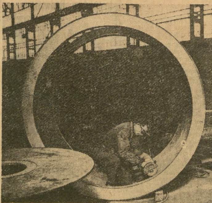
Fragment radioteleskopu
