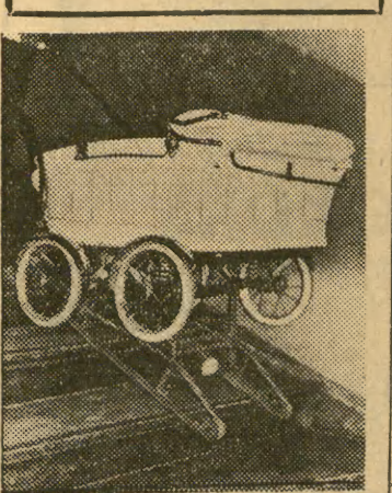
Dodatkowe „podwozie” z ruchomymi pasami jest tak skonstruowane, że wózek zjeżdżając po schodach utrzymuje pozycję poziomą.
