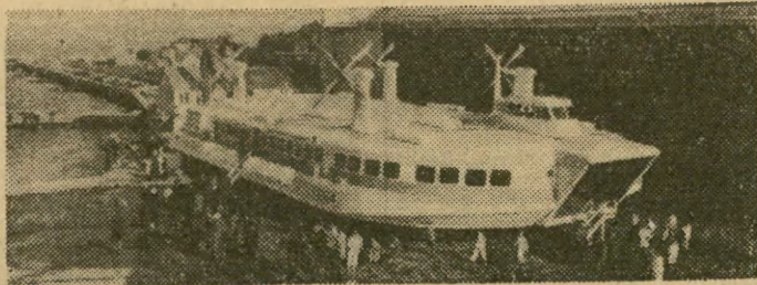
Brytyjskie zakłady British Hovercraft Corporation przystąpiły do prób technicznych z poduszkościvem typu SRN-4. Jest to największy z dotychczas wyprodukowanych poduszkościvów. O ile próby wypadną pomyślnie, wehikul od przyszłego roku zacznie regularną „żeglugę” między Wielką Brytanią i Francją zabierając jednorazowo 609 pasażerów lub 254 pasażerów i 30 samochodów. Poduszkościv SRN-4 waży 165 ton. Przesmyk kanatu La Manche oddzielający Francję od Wysp Brytyjskich będzie przebywać, w ok. pół godziny. CAF Telefoto
