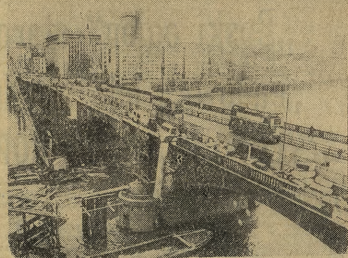
Na zdjęciu: jednocześnie z robót 134-letniego mostu londyńskiego, trwa budowa nowoczesnego, 6-pasmowego mostu. Stary most podzielono na blisko
