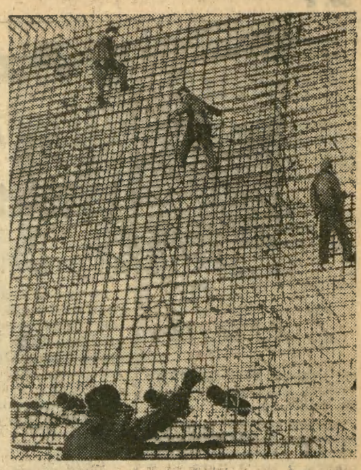
Ta „pajęcza sieć” ze stalowych prętów — to konstrukcja jednej ze ścian budynku kolejowej elektrowni atomowej, budowanej w ZSRR. CAF — TASS
