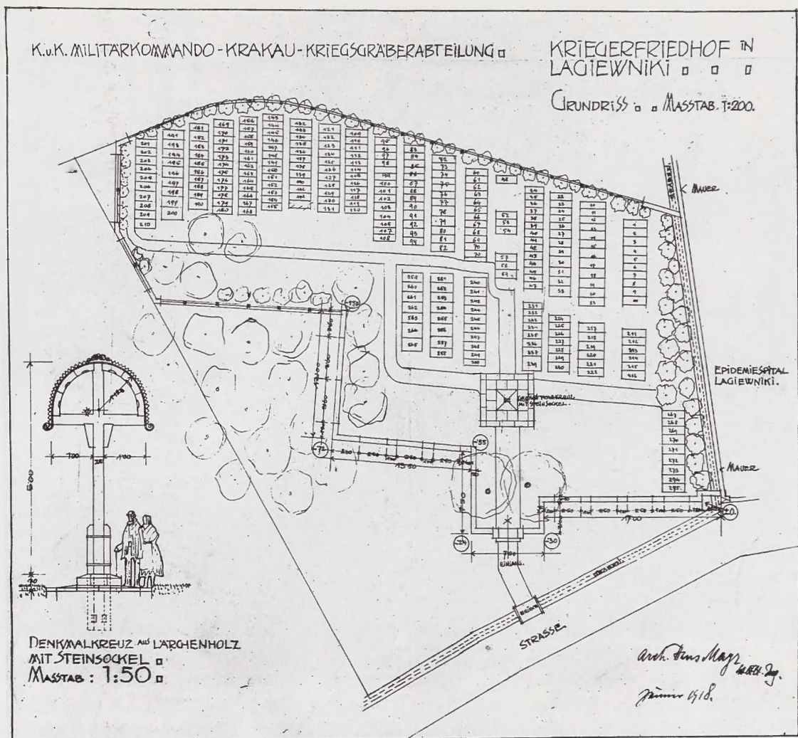
10. Hans Mayr, projekt cmentarza w Łagiewnikach, rysunek tuszem na kalce, styczeń 1918
