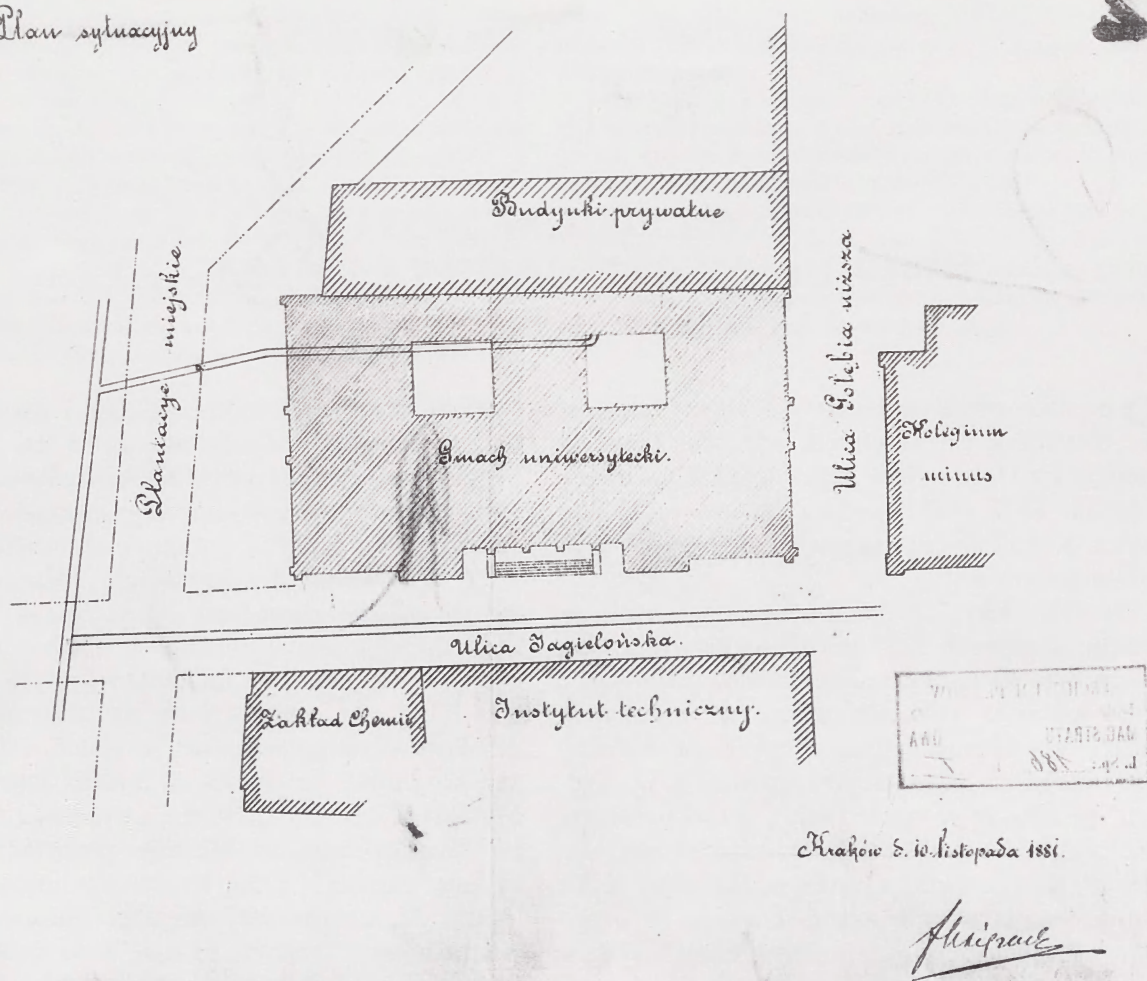
1. Plan sytuacyjny gmachu uniwersyteckiego z roku 1881 (z fasadą od ul. Jagiellońskiej)
