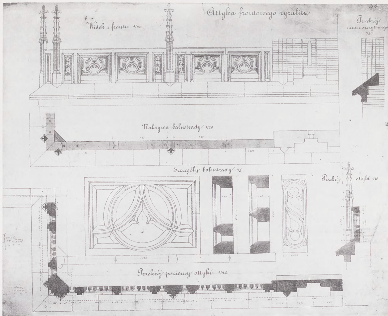
3. Projekt detalu kamiennego z fasady Collegium Novum (z czasów budowy gmachu)
