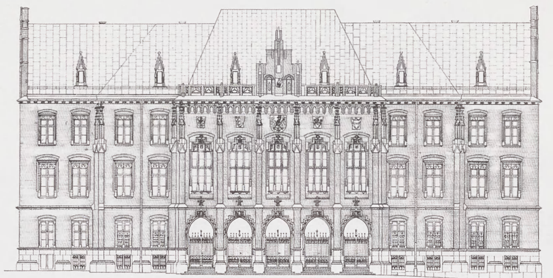
2. Fasada Collegium Novum (wg pomiaru sporządzonego w r. 1975 przez Miejskie Przedsiębiorstwo Geodezyjne w Krakowie)
