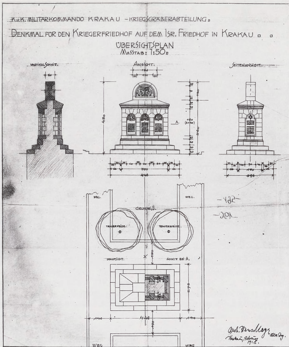
12. Hans Mayr, projekt żydowskiego cmentarza wojennego w Krakowie, rysunek tuszem na kalce, luty 1918
