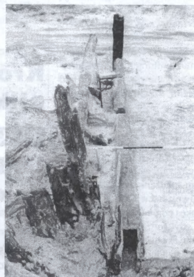
3. Pale i belki z konstrukcji pomostu - belki mają długość ok. 6-7 metrów (fot. D. Rozmus)
