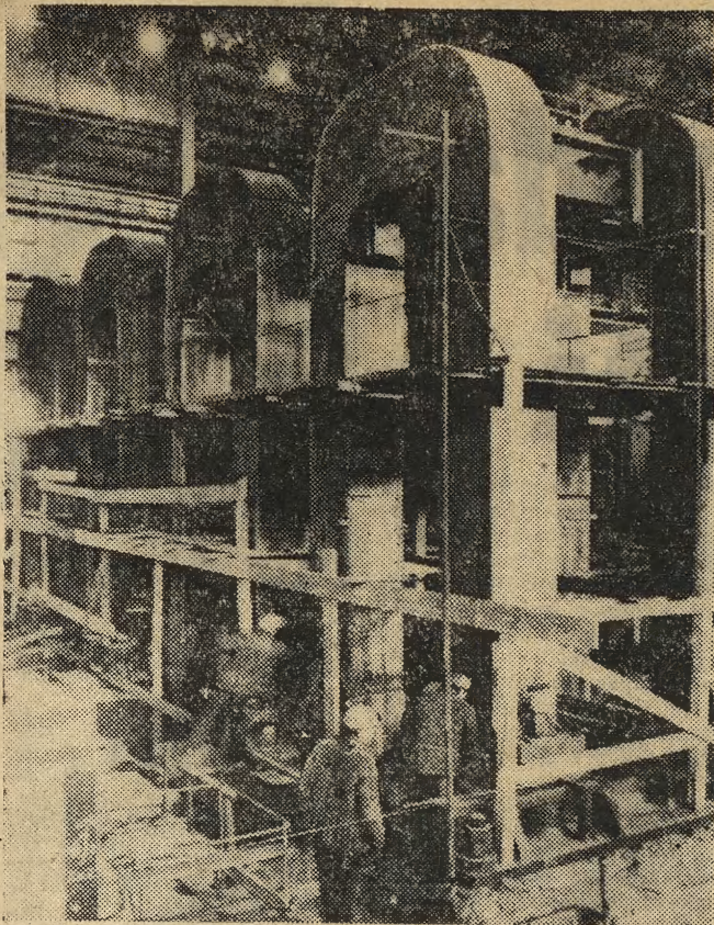
Gotowe są już potężne stojaki, na których również „mostostalowcy” zamontują walcarkę 4-klatkową dla blach karoseryjnych.
