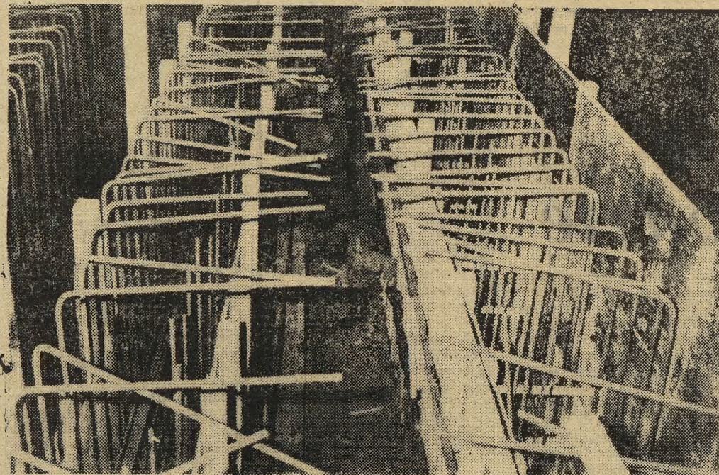
Zbrojenie fundamentów technicznych i technologicznych pod urządzenia do wyżarzania blachy.
