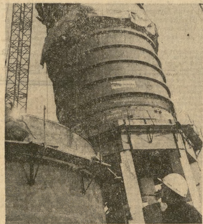
Montaż kolumny destylacji próżniowej gdańskiej rafinerii. Będzie miała ona niebagatelną wysokość — 53 m.
