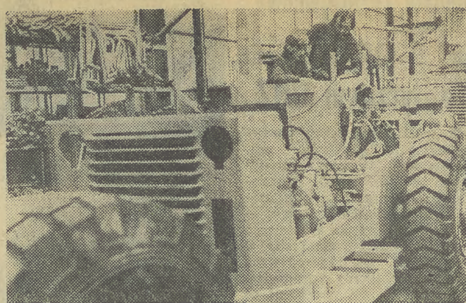
Fabryka Maszyn Budowlanych FADROMA we Wrocławiu, jest znanym producentem różnego rodzaju ładowarek. Powstają tu także ciągniki do górniczych wozów wiertniczych i kotłowych, a w kooperacji ze szwedzką firmą Kockums, wytwarzane są 17-tonowe wywrotki K-412. Na zdjęciu: montaż ładowarek L-2 na nowoczesnej taśmie produkcyjnej. CAF — Hawalej
