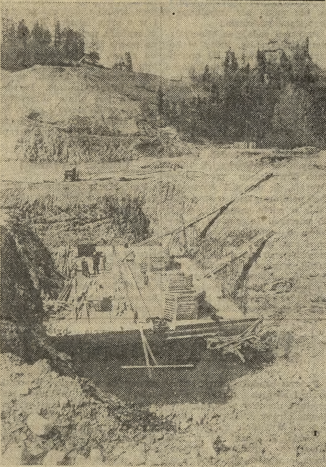
Pierwsze fundamenty obiektów wodnych budowane w sąsiedztwie zamku w Niedzicy.
