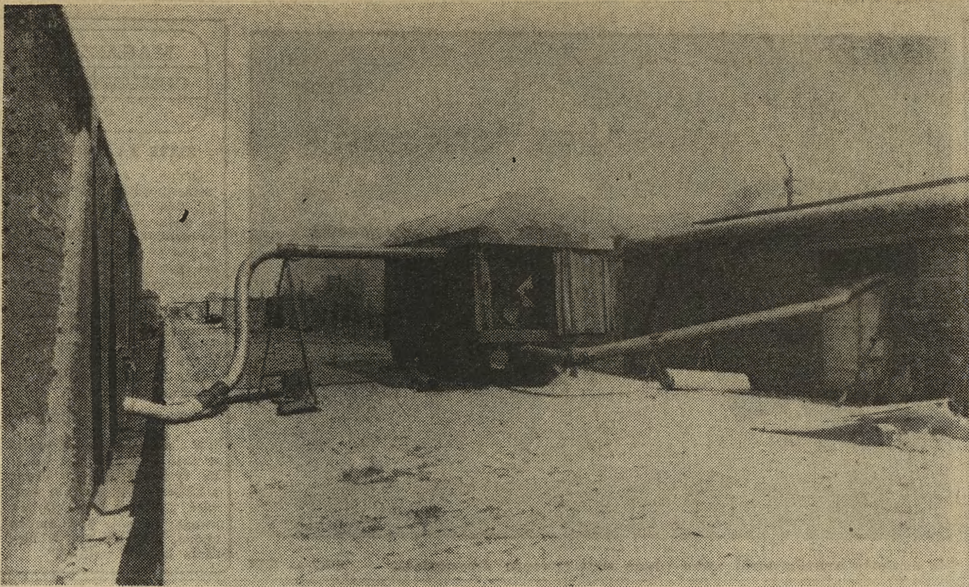
W Żurawicy, przy pomocy przenośników elektropneumatycznych zboże bezpośrednio przesypuje się z radzieckich do polskich wagonów.
