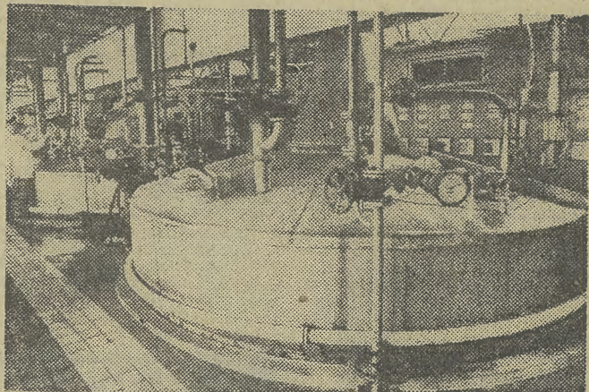
Fragment hali ze zbiornikami fermentacyjnymi o pojemności 118 m sześci.
