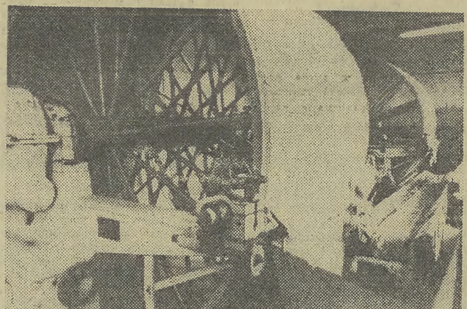
Filtry zagęszczające mleczko drożdżowe do stałej konsystencji. Fot. JADWIGA RUBIS
