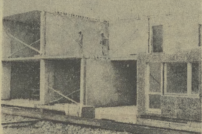
Z takich gotowych, prefabrykowanych płyt montuje się domy. Na pierwszym planie zewnętrzna ściana z gotowymi drzwiami i oknem. Widoczna elewacja z witrażem.
