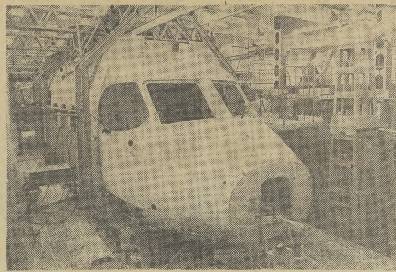
Zgodnie z umową polsko-radziecką w mieleckiej Wytwórni Sprzętu Komunikacyjnego trwają prace nad uruchomieniem produkcji samolotu pasażerskiego AN-28, w oparciu o dokumentację z biura konstrukcyjnego Olega K. Antonowa. Na zdjęciu: montaż kadłuba samolotu.
