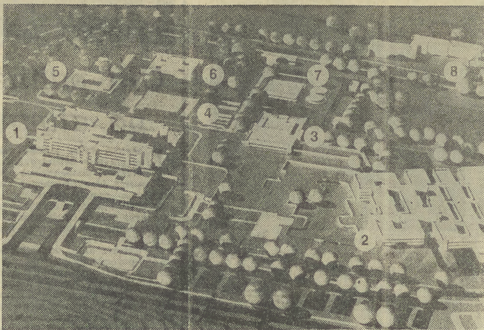
1. Szpital ginekologiczno-położniczy, 2. Szpital pediatryczny, 3. Kuchnia, 4. Pralnia, 5. Anatomia patologiczna, 6. Warsztaty i magazyna, 7. Centrala techniczna, 8. Hotel.
