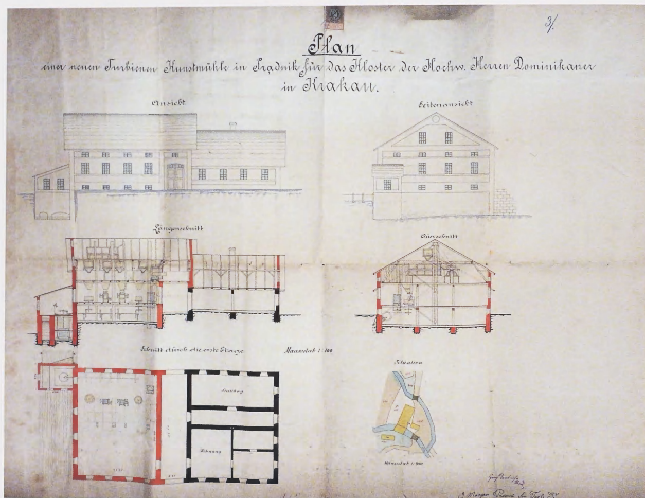
17. Projekt młyna dominikańskiego na Prądniku Czerwonym z 1890 r. Repr. ze zbiorów ADKr, sygn. Kr 1043
