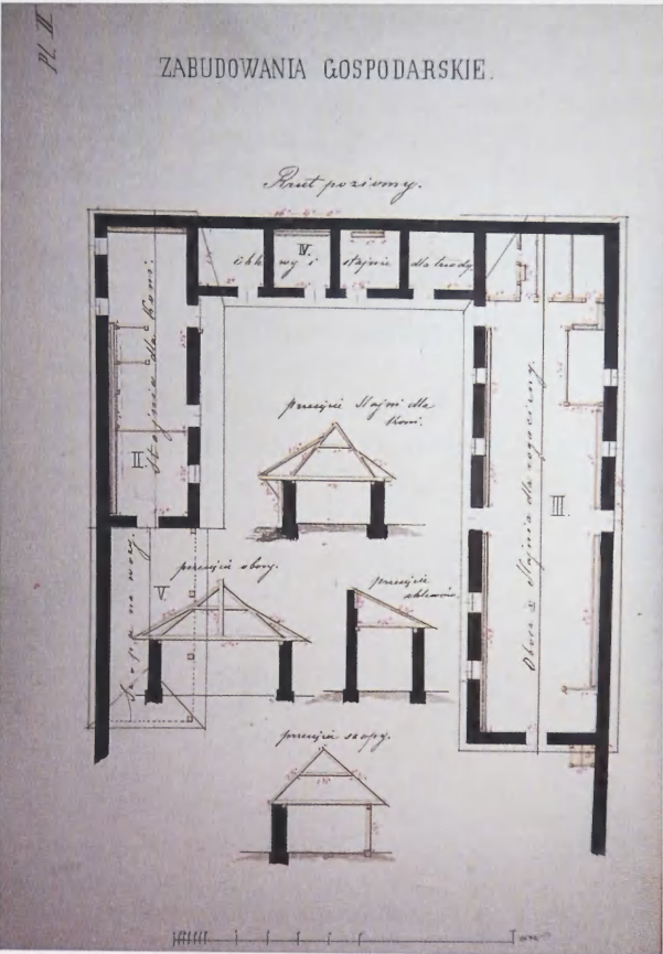
9. Folwark dominikański na Prądniku Czerwonym. Inwentaryzacja zespołu zabudowań gospodarczych oo. dominikanów na Prądniku Czerwonym z 1865 r. Repr. ze zbiorów ADKr, sygn. Kr 783
