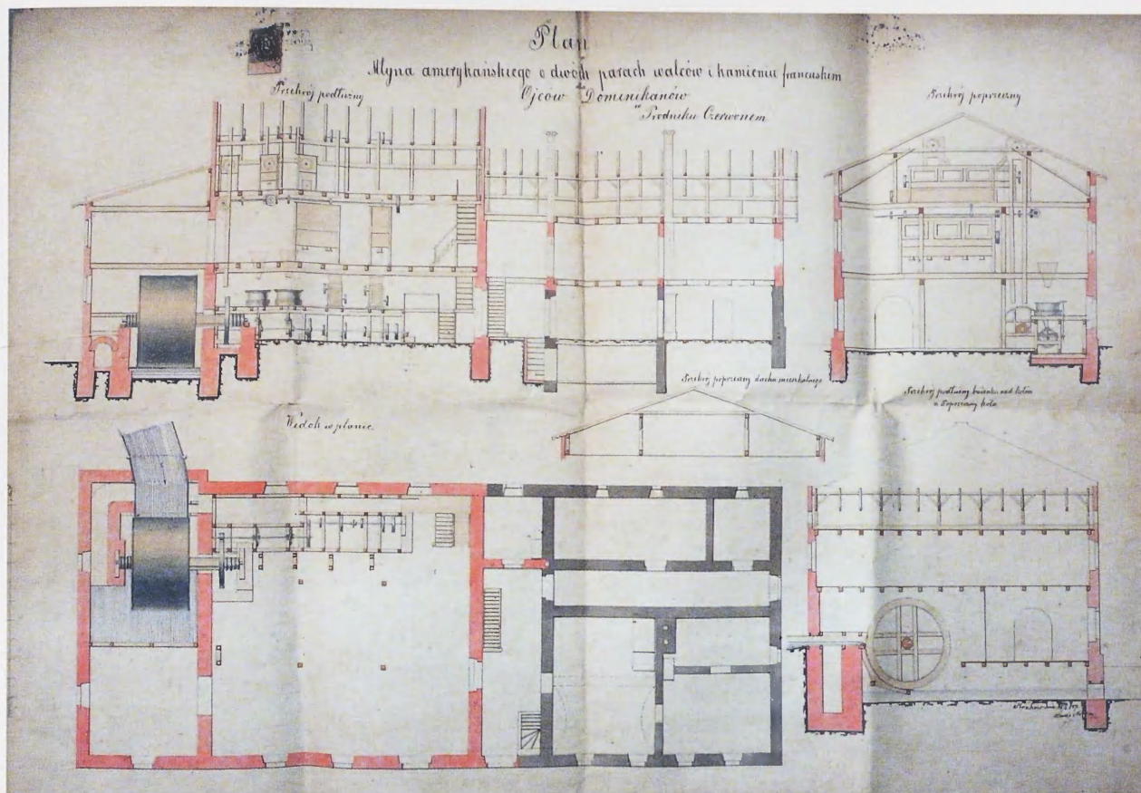
16. Projekt młyna dominikańskiego na Prądniku Czerwonym z 1887 r. Repr. ze zbiorów ADKr, sygn. Kr 1043
