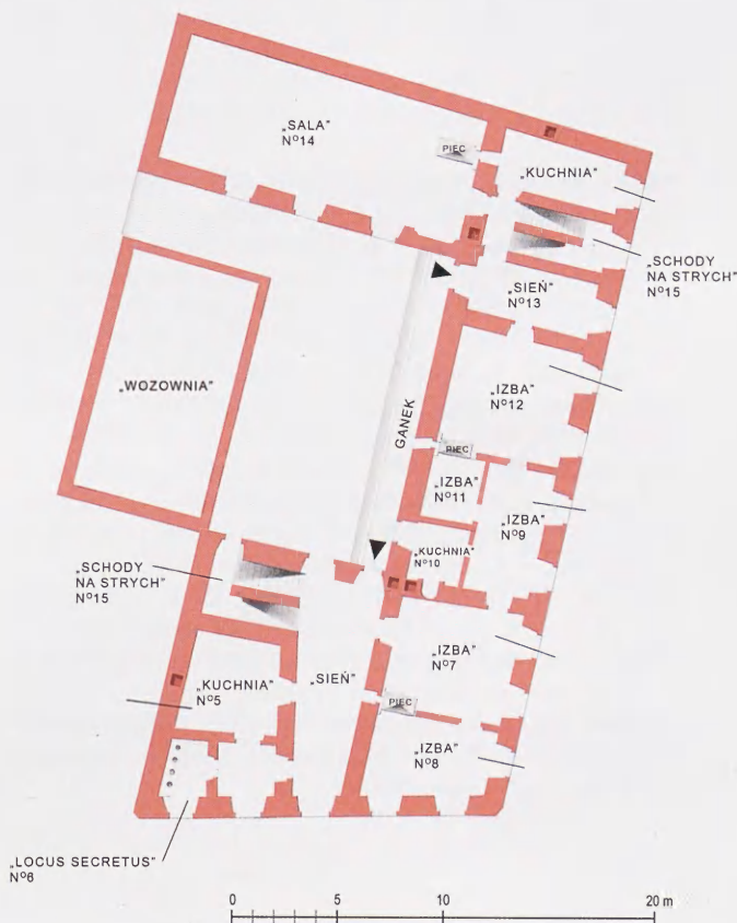
8. Lazareet garnizonu krakowskiego (dziś przy ul. Siennej 16 / ul. Świętego Krzyża 2). Rekonstrukcja stanu z 1792 r. – rzut parteru. Opracowano na podkładzie planu z 1801 r. Za: ANK, Archiwum planów Budownictwa Miejskiego, sygn. ABM, Plany architektoniczne, dom ul. Sienna 16, plany 1–5
