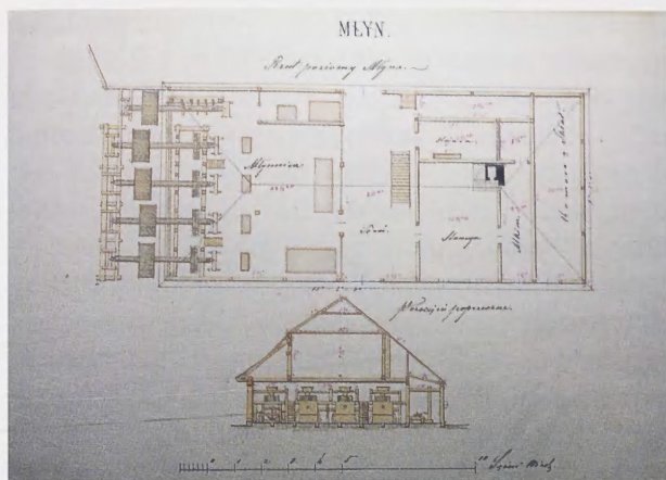
20. Młyn dominikański na Prądniku Czerwonym: rzut poziomy i przekrój poprzeczny. Inwentaryzacja z 1865 r. Repr. ze zbiorów ADKr, sygn. Kr 783
