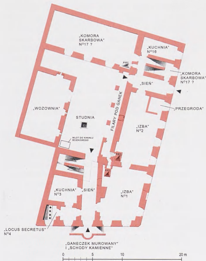
8. Lazareet garnizonu krakowskiego (dziś przy ul. Siennej 16 / ul. Świętego Krzyża 2). Rekonstrukcja stanu z 1792 r. – rzut parteru. Opracowano na podkładzie planu z 1801 r. Za: ANK, Archiwum planów Budownictwa Miejskiego, sygn. ABM, Plany architektoniczne, dom ul. Sienna 16, plany 1–5
