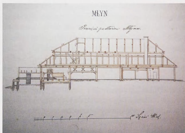
21. Młyn dominikański na Prądniku Czerwonym: przekrój podłużny. Inwentaryzacja z 1865 r. Repr. ze zbiorów ADKr, sygn. Kr 783
