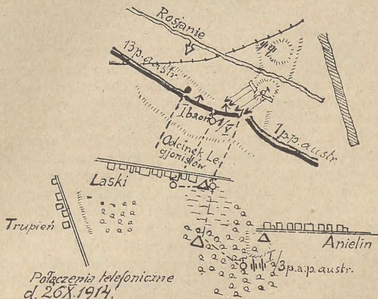
Rys. 15. Połączenia telefoniczne na pozycjach pod Laskami 26.X.1914.
