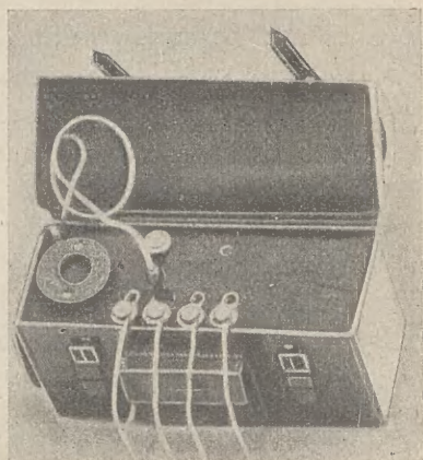
Rys. 6. Telefon polowy otwarty.
