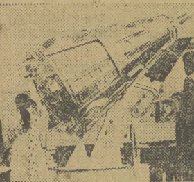
2. Sputnik II
