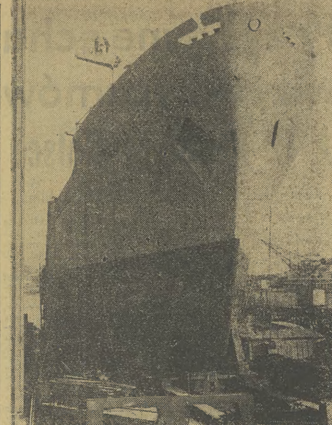
W dniu 7 stycznia br. odbyło się w Stocznii Im. A. Warskiego w Szczecinie pierwsze w tym roku wodowanie statku. Zwodowany został drobniowiec motorowy typu B-455, któremu nadano imię „Gdynia II”. Jest to 142 jednostka zwodowana w tej Stoczni po wojnie. Nowy statek jest przeznaczony dla Polskiej Żeglugi Morskiej w Szczecinie i pływac będzie na linii zachodnio-afrykańskiej, tej samej, na której pływa M/S „Kraków”. Na zdjęciu: „Gdynia II” na chwilę przed wodowaniem.
