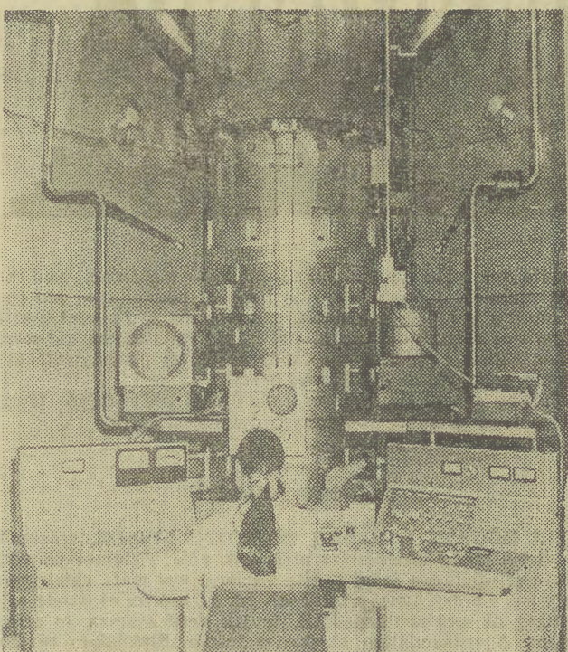
NAJWIĘKSZY NA ŚWIECIE MIKROSKOP ELEKTRONOWY. Oibrymi 3 000 000-woltowy mikroskop elektroniczny zbudował po 2 latach prób naukowych z uniwersytetu w Osace, przy współdziałaniu firmy Hitachi Limited. Prace badawcze i produkcja pochłonęły ponad 1,5 mln dolarów USA. Mikroskop może powiększać do 100 000 razy. Znajdzie zastosowanie do badania komórek raka oraz wirusów.
