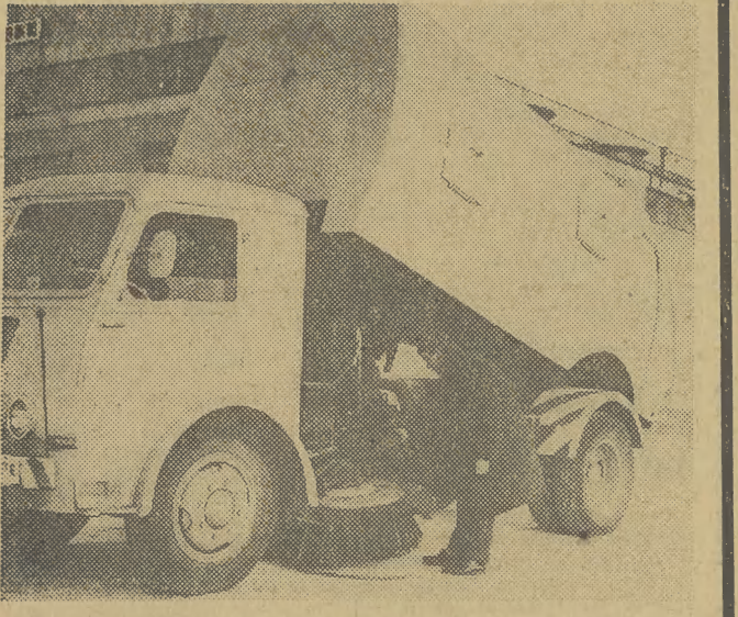
Wytwórnia Urzędzeń Komunalnych „Wuko” w Łodzi skonstruowała i wykonała prototyp ulicznej zamlatarki samobieżnej. Zamlatarka wyposażona jest w komplet szczotek stalowych, które wmiatają śmieci pod samochód, ślad szczotki znajdująca się pod samochodem podnosi je i podtrzymuje pod kolektor śmieci, którym dostają się one do wnętrza zbiornika. Aby zamlatanie odbywało się bezpylnie, nowy samochód asenizacyjny posiada rozpylacze, które pod ciśnieniem trzech atmosfer rozpylają wodę tworząc mgłę wokół szczotek. Zamlatarka porusza się w zależności od potrzeb tj. stopnia zanieczyszczenia jezdni z szybkością 4-20 km/godz. czyszcząc pas szerokości 2,5 m. Na zdjęciu: mgr inż. Konrad Kobryń przy prototypie zamlatarki. CAF — fot. Rozmysłowicz
