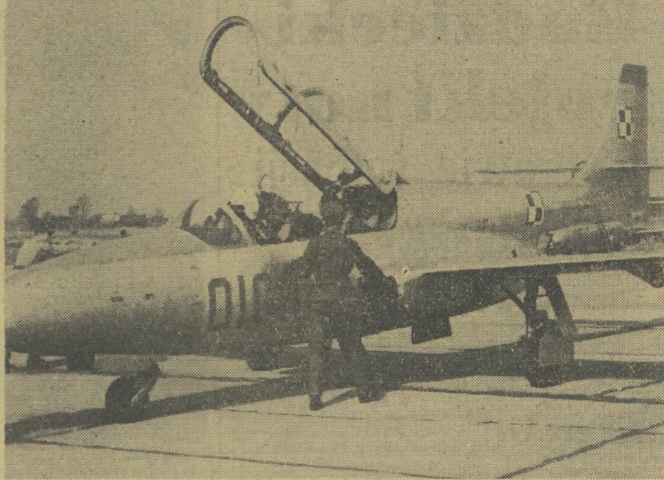
PIERWSZE SAMOLOTY ODRZUTOWE POLSKIEJ KONSTRUKCJI Na zdjęciu: przygotowana do startu samolotu odrzutowego polskiej produkcji TS-11 „Iskra”. CAF — fot. Matuszewski
