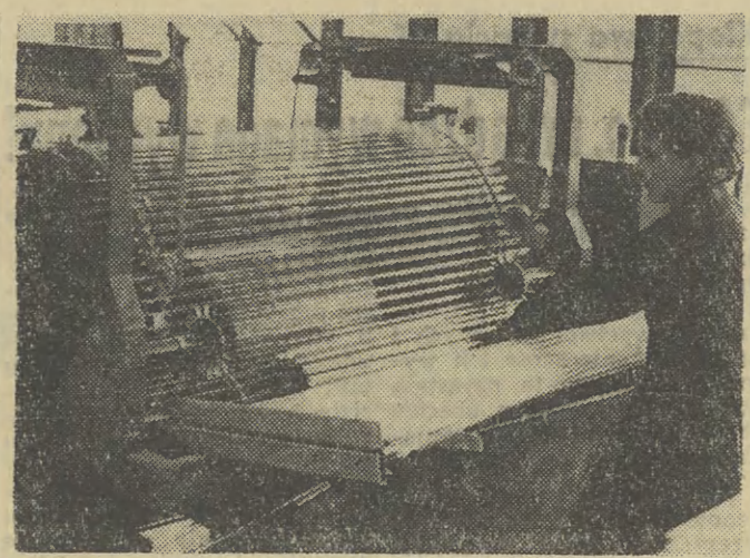
Krośnieńskie Huty Szkła są znanym wytwórcą wyrobów z różnych rodzajów szkła technicznego. Na zdjęciu: maszyna do obcinania i zatapiała na brzegów rurek ze szkła neutralnego. CAF — Kwiatkowski
