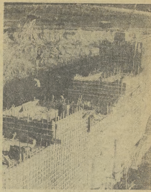
Na Włókno w rejonie Beska dobiega końca budowa zapory wodnej. Spierająca woda tworzy zbiornik retencyjny, który pozwoli na znaczną poprawę w gospodarowaniu zasobami wodnymi w tym rejonie. Wiosną zniweluje skutki obfitych opadów, zalewających grunty orne, latem uzupełni występujący niedobór wody. Poza tym ze zbiornika popłynie woda do znanych uzdrowisk w Rymanowie i Iwoniu. (CAF — Łokaj)
