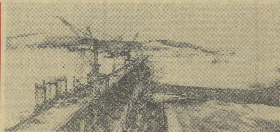
ZSRR. Pierwsze trzy agregaty o mocy 240 MW każdy Ust-Dimskiej Elektrowni Wodnej. Na zdjęciu: panorama Ust-Dimskiej Elektrowni Wodnej. CAF — TASS
