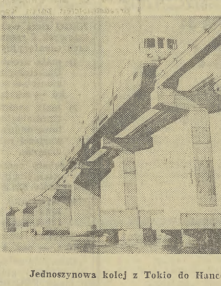
Jednoszynowa kolej z Tokio do Haneda
