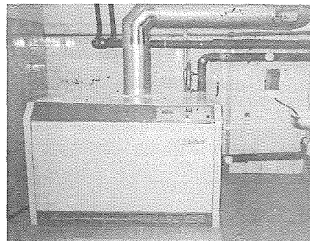
Piec gazowy w harbutowickiej szkole
