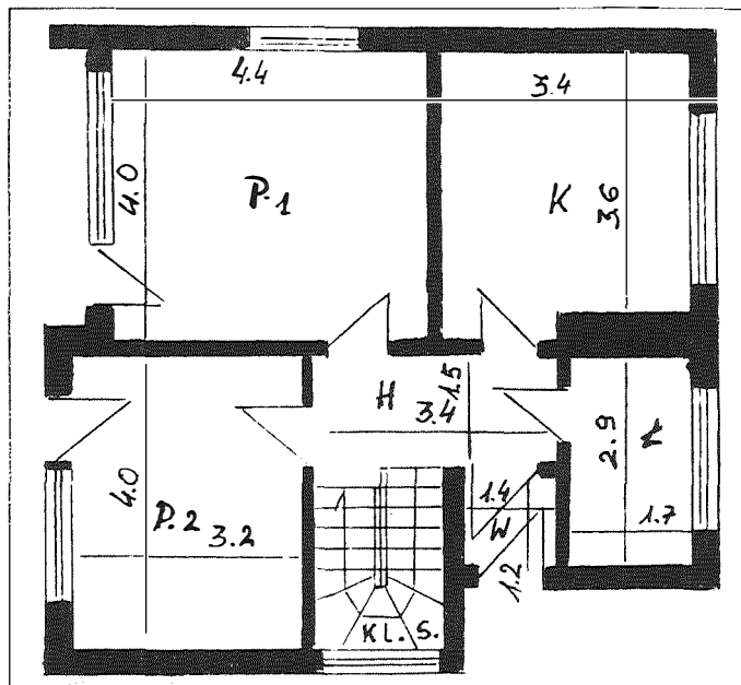
Rys. 1 RZUT PARTERU
