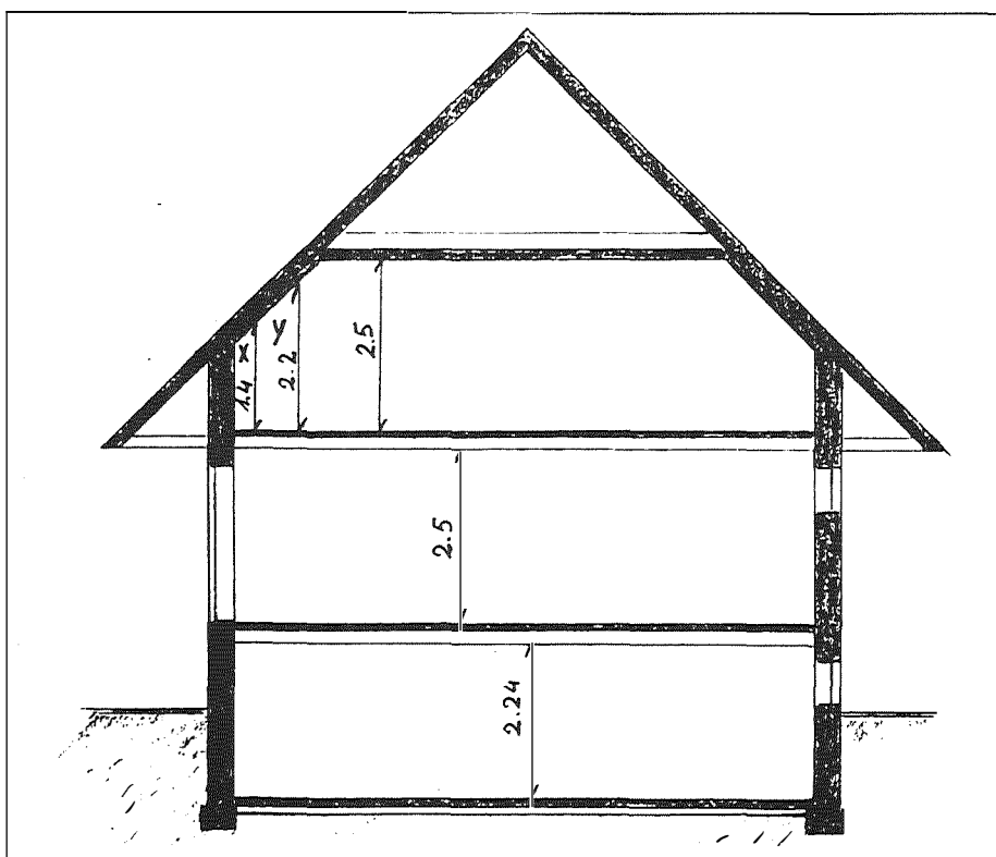
Rys. 3 PRZEKRÓJ
