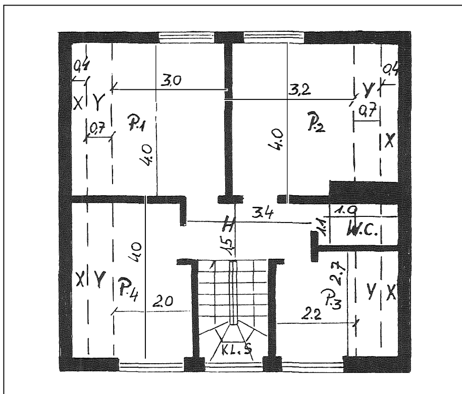
Rys. 2 RZUT PODDASZA
