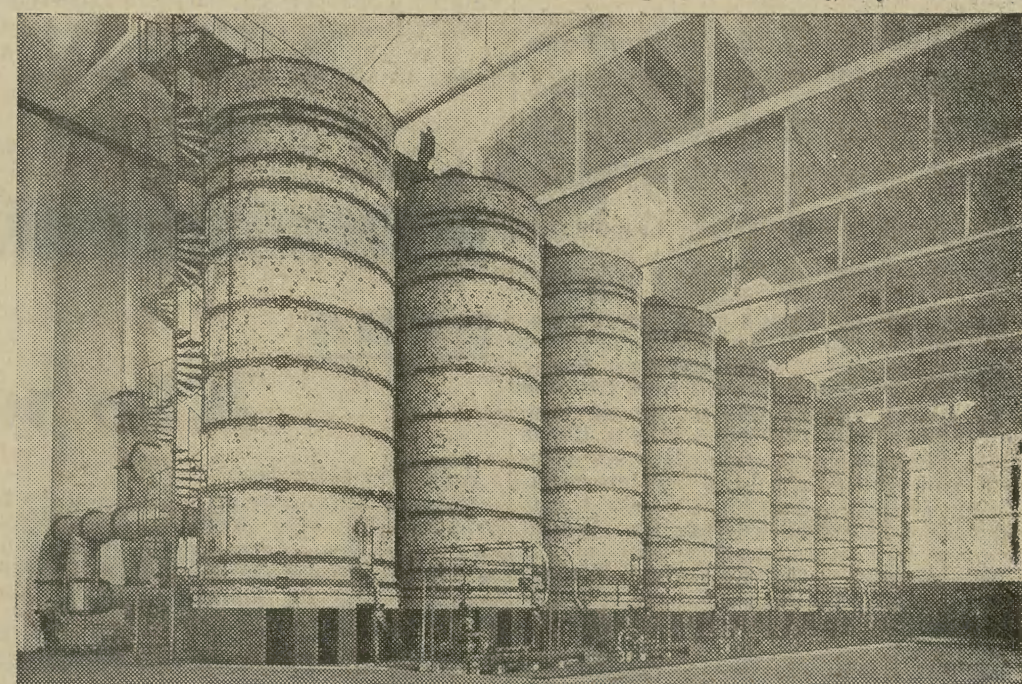
Wieże absorbcyjne dla otrzymywania kwasu azotowego w Państw. Fabryce Związków Azotowych w Mościcach, zbudowane według systemu P. Prezydenta R. P. prof. I. Mościckiego.
