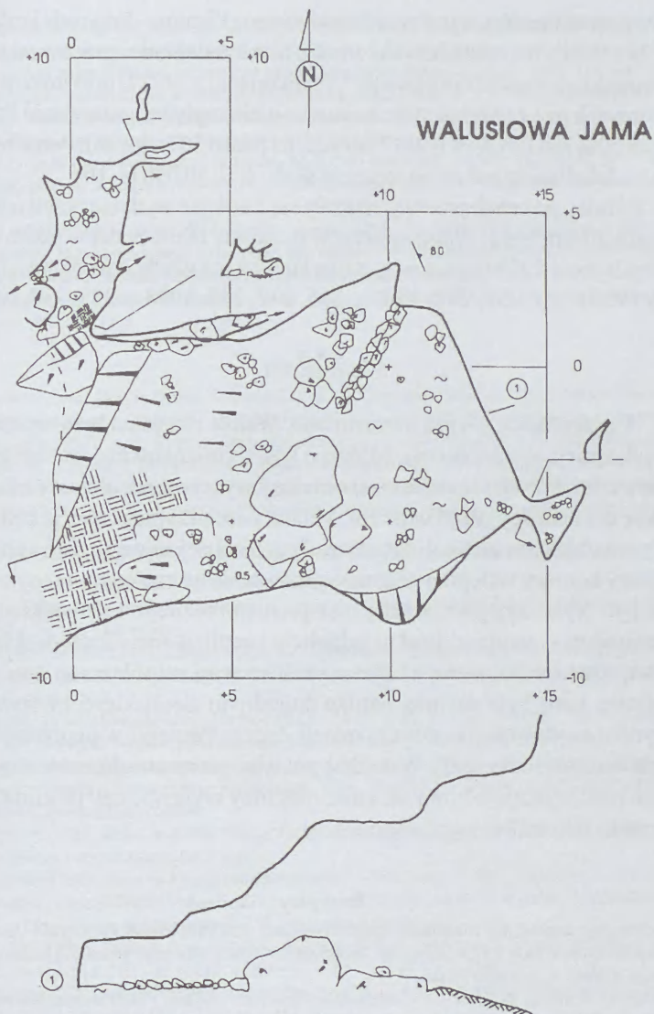
Plan jaskini Walusiowa Jama - A. Amirowicz (pomiary: A. Amirowicz, K. Dziubek, M. Gradziński) Pieniny - przyroda i człowiek , t. 3, 1995, s. 28 (Uwaga przekrój jaskini jest odwrócony)
