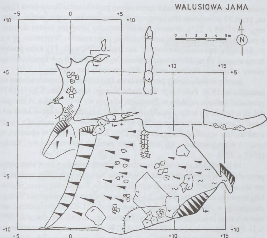
Plan jaskini Walusiowa Jama - A. Amirowicz, M. Gradziński (pomiar: A. Amirowicz, K. Dziubek, M. Gradziński 22. 04. 1993 r.) Amirowicz i in. mat. arch.1993
