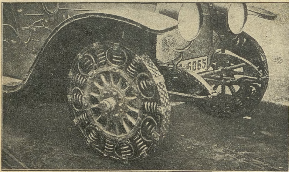
Samochód na kołach sprężynowych zamiast opon.
