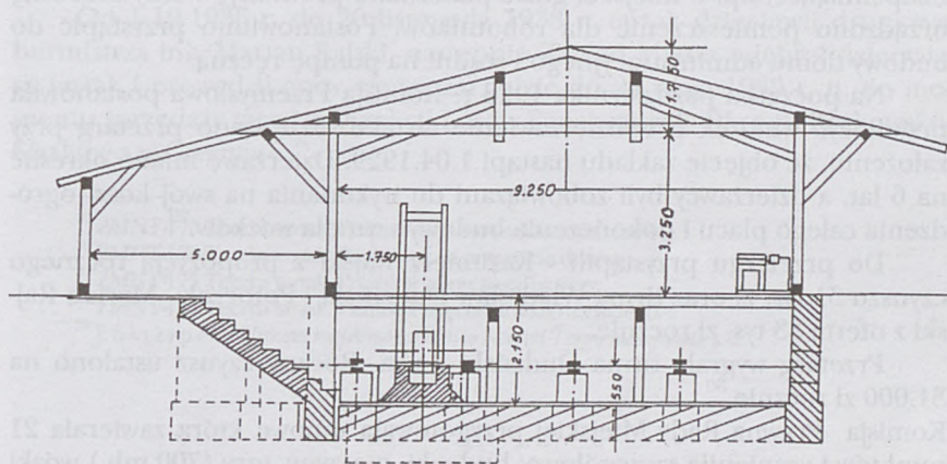
Przekrój poprzeczny hali tartaczanej stan z 1927 r., rys. A. Lohn, na podstawie planu firmy „Unia” z Bydgoszczy.
