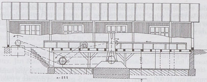
Przekrój podłużny hali tartaczanej stan z 1927 r., rys. A. Lohn, na podstawie planu firmy „Unia” z Bydgoszczy.
