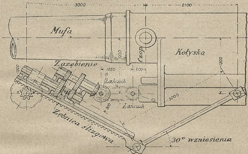
Przyrząd celowniczy o 2-ch prędkościach.
