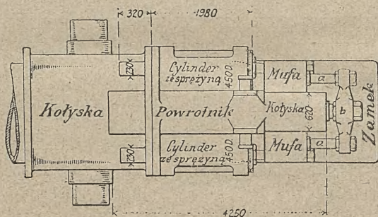
Kolyska, w której jest umieszczona armata z cylindrami hamulca i z powrotnikiem.
