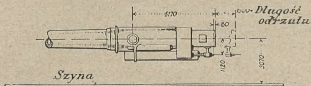
Całość urządzenia hamującego.
