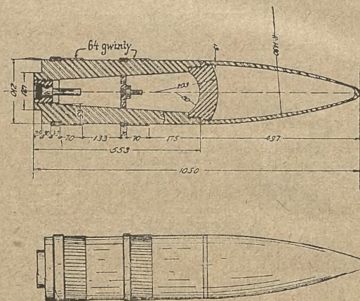
Pocisk gwintowany Borty swoim kapturem czepiec przepona i dwoma pierścieniami
