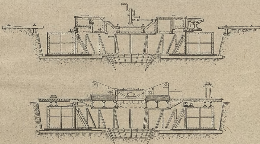
Ustawienie Berty w lesie Châtelet — budowa dolna ze stali i betonu dźwiga za pośrednictwem korony na kulach 20 cm. obracającą się płat formę armaty.
