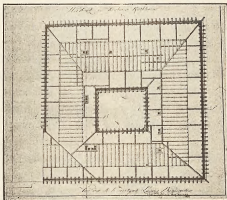
Fig. 22. Wiązanie dachowe ratusza na spichlerzu.
