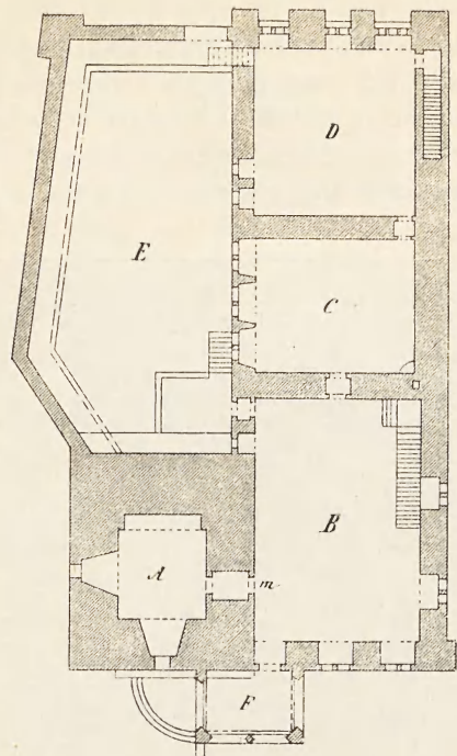
Fig. 20. Rzut poziomy parteru pierwotnego ratusza (podług Essenweina).
