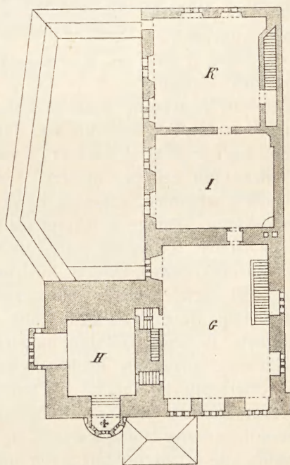
Fig. 21. Rzut poziomy I. piętra pierwotnego ratusza (podług Essenweina).
