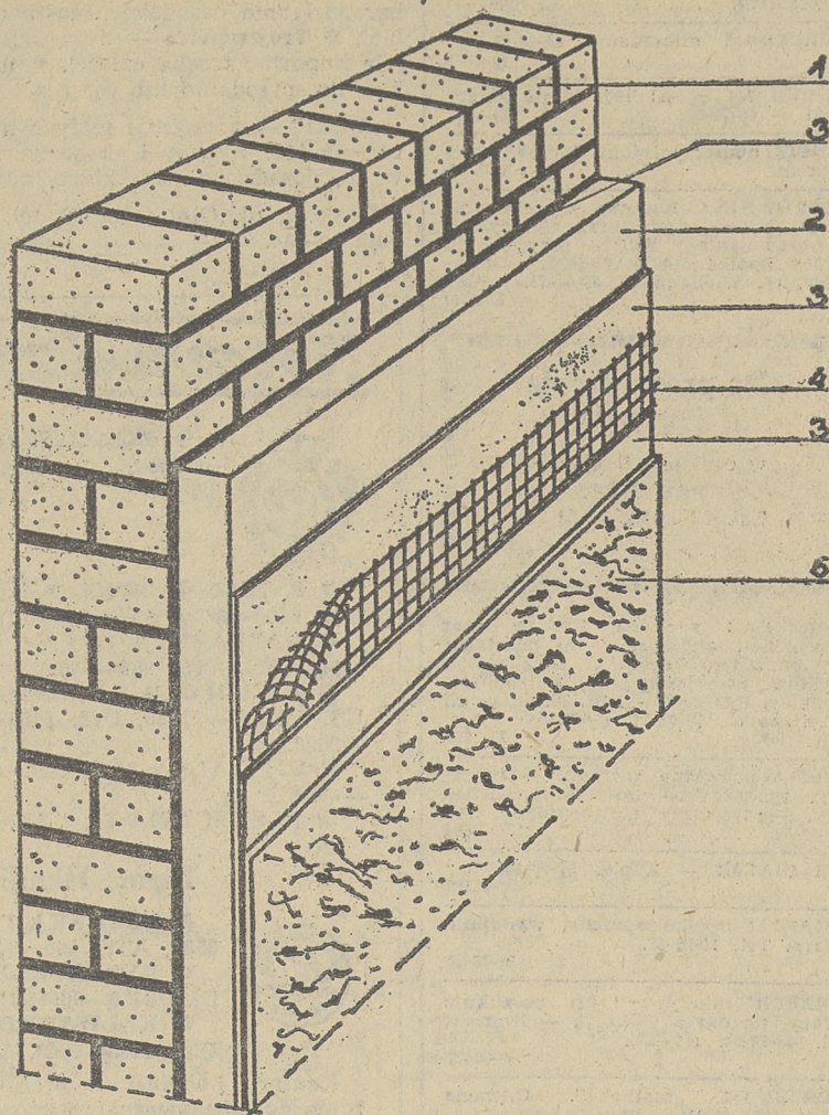
1. Sciana nośna. 2. Styropian. 3. Masa podkładowa klejąca. 4. Siatka z włókna szklanego. 5. Tynk szlachetny cienkowarstwowy.
