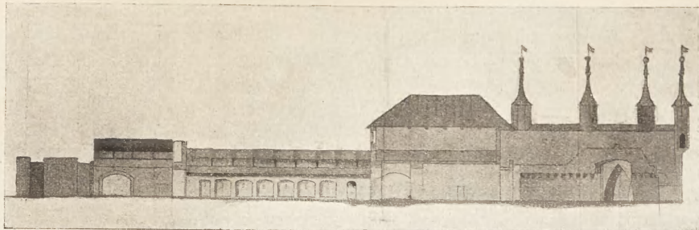
Fig. 19. Przekrój podłużny barbakanu wraz ze zburzoną szczyłą. Z archiwum Budownictwa miejskiego.
