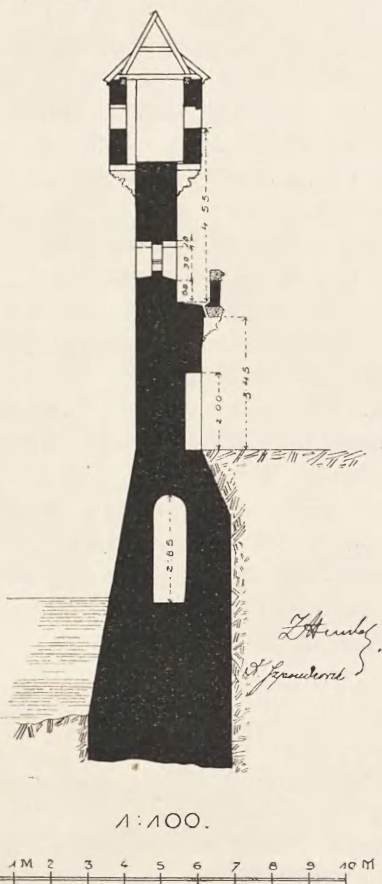
Fig. 18. Przekrój poprzeczny barbakanu od strony miasta.
