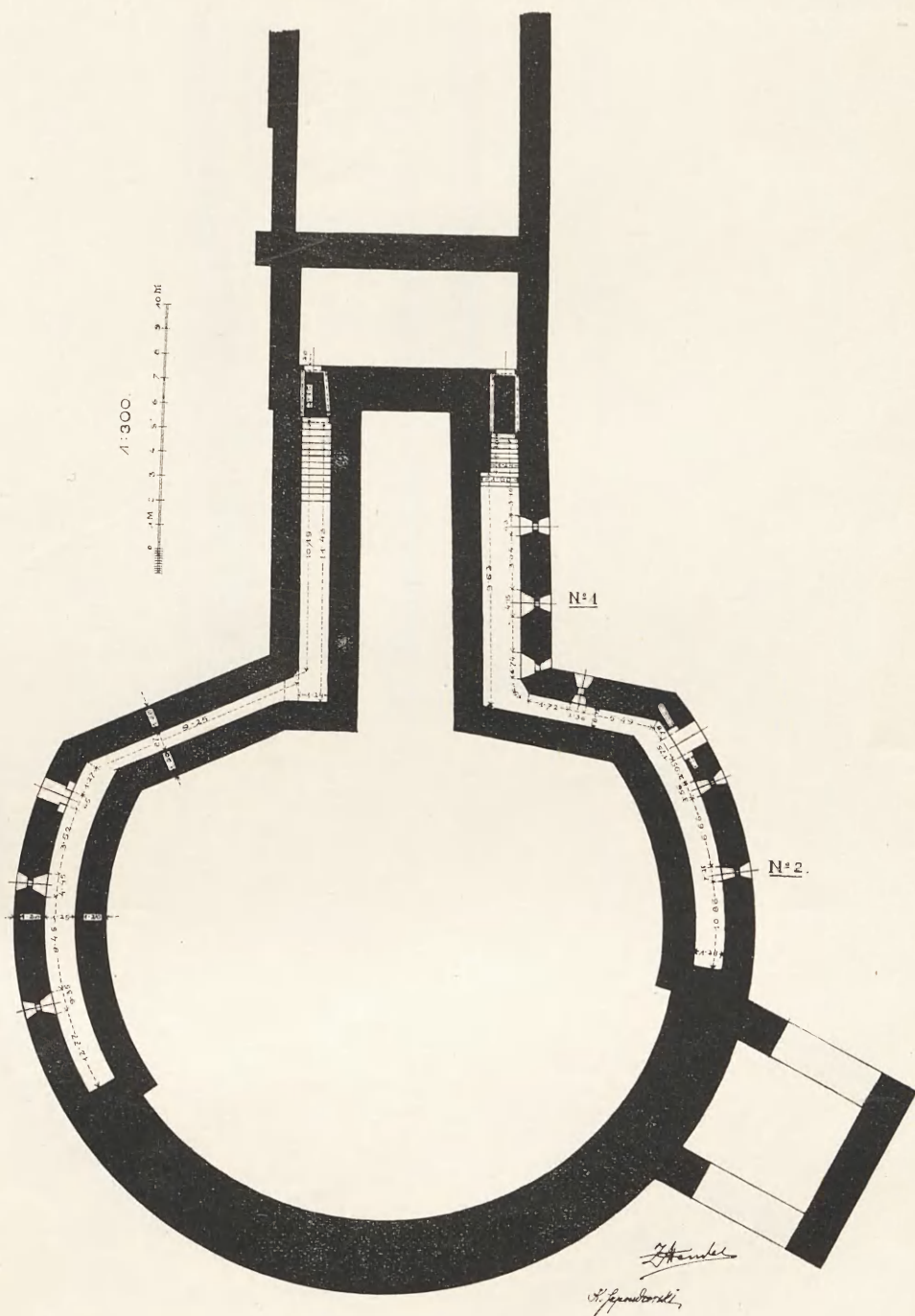
PRZEKRÓJ PODŁUŻNY PRZYZIEMIA BARBAKANU.
