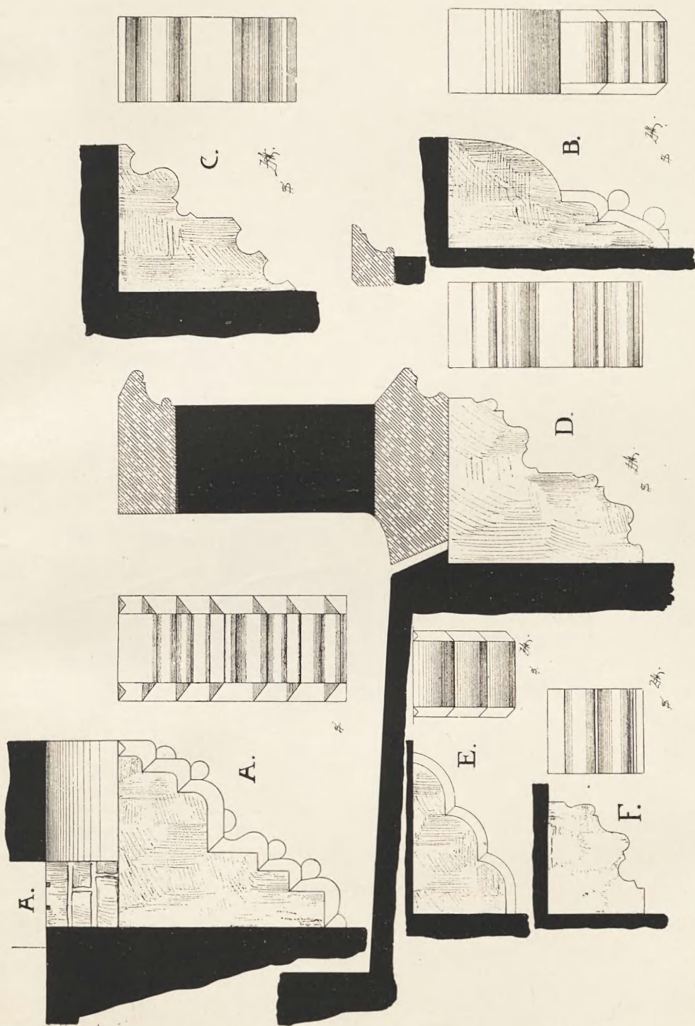
PRZEKRÓJ POPRZECZNY KONSOL BARBAKANU.
