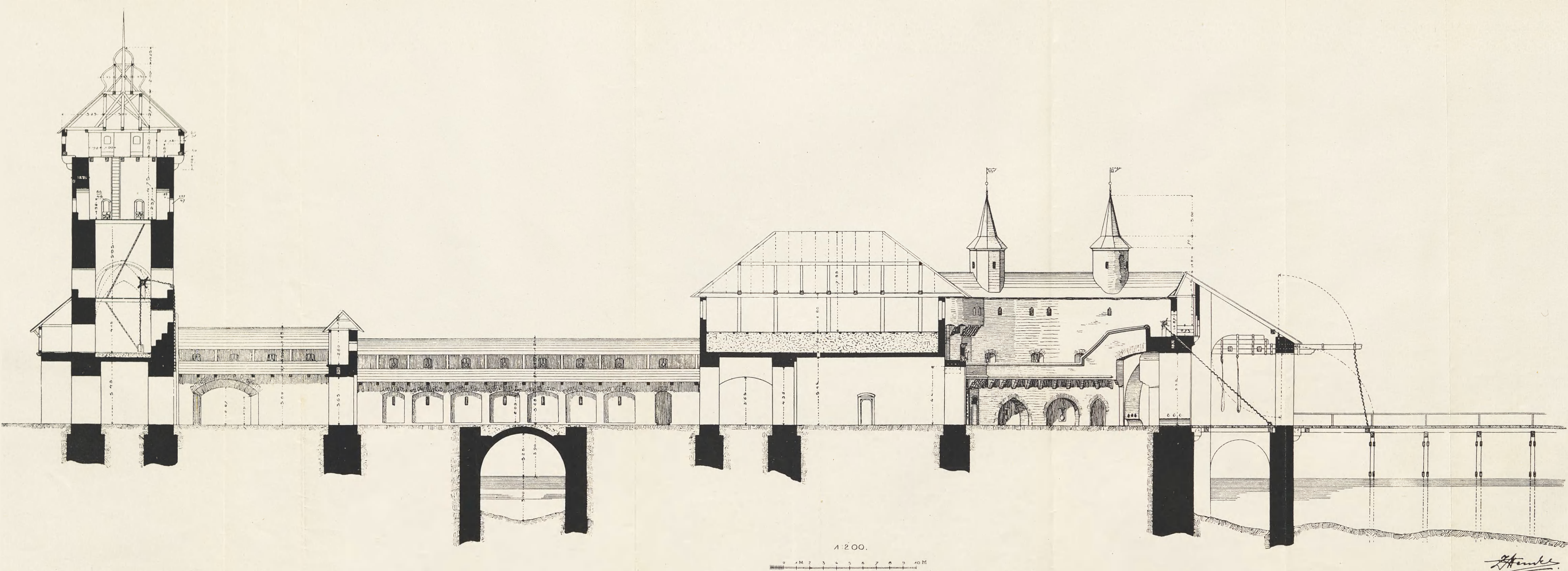
PRZESZKÓJ PODŁUŻNY: BASZTY FLORYAŃSKIEJ, SZYI ŁĄCZĄCEJ TĘ BASZTĘ Z BARBAKANEM I BARBAKANU.
