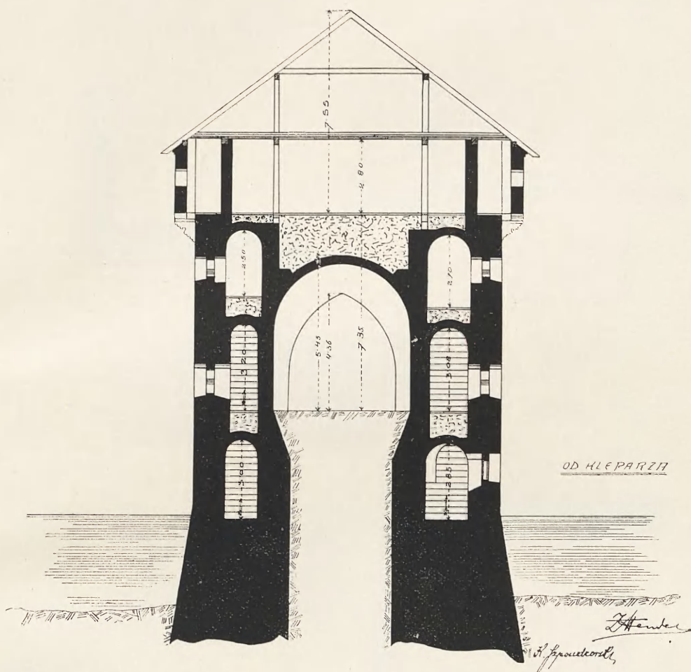
PRZEKRÓJ POPRZECZNY SZYI BARBAKANU.
