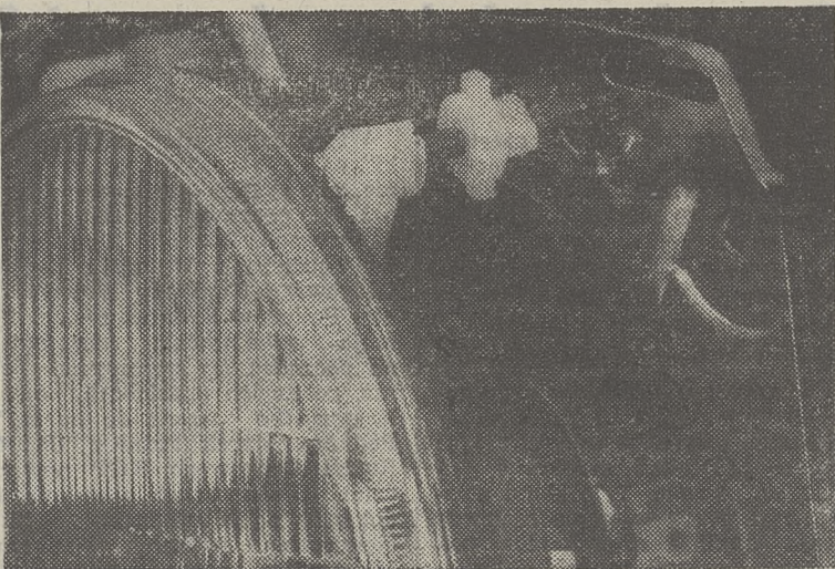
Zerwana śruba w „podróbce” stanowi efekt testu z którym bez trudu dają sobie radę reflektory firmowe.
