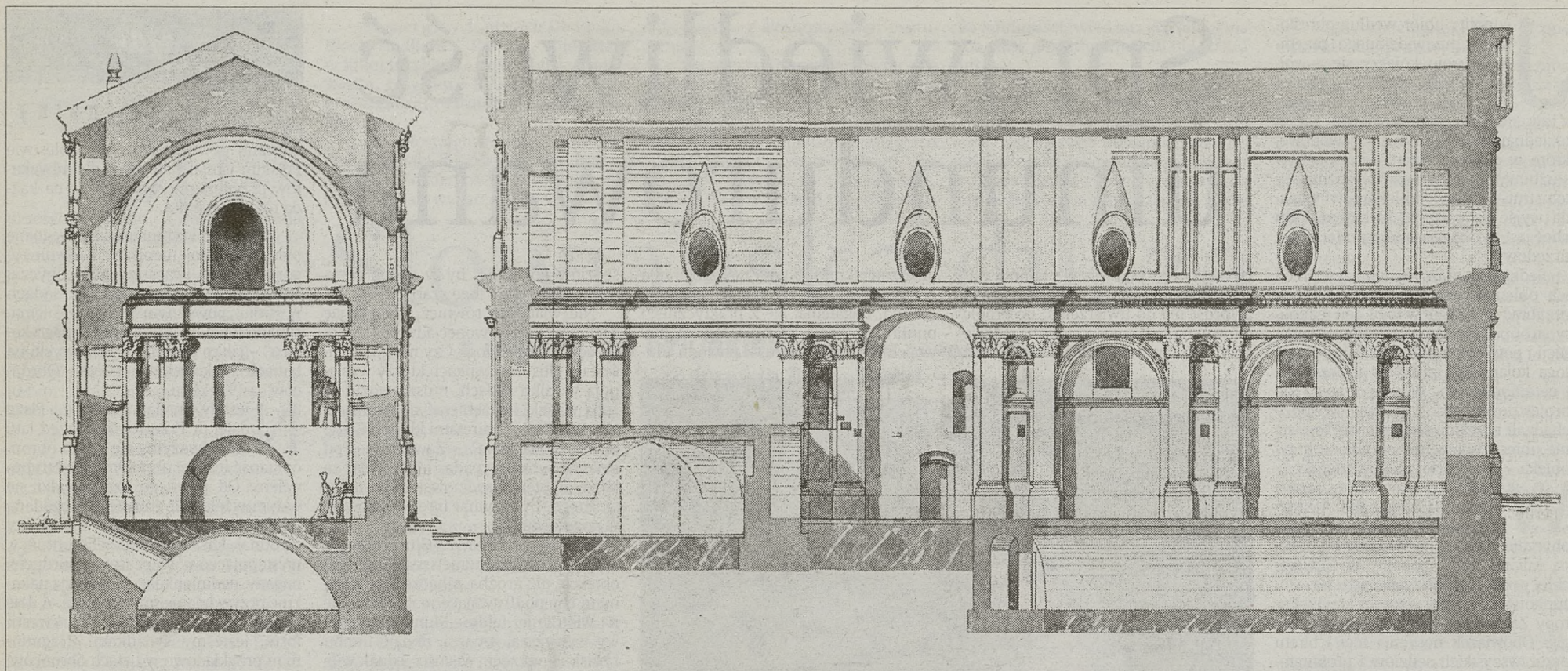
Kościół św. Agnieszki – przekrój poprzeczny i podłużny
