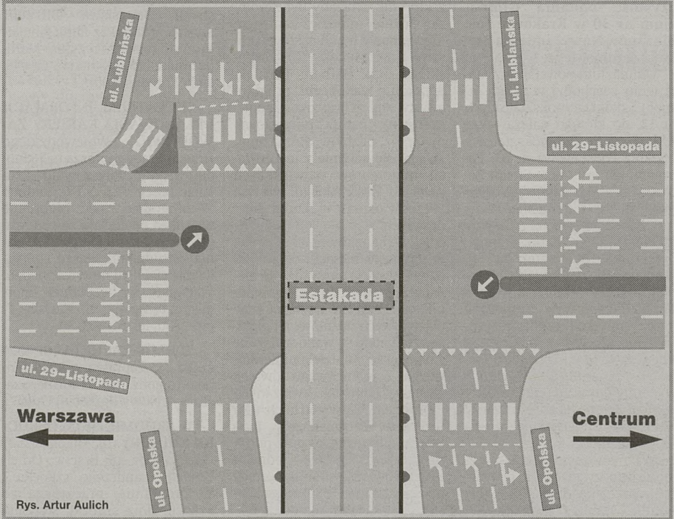
Na skrzyżowaniu al. 29 Listopada z ul. Opolską i Lublańską wprowadzono nową organizację ruchu
