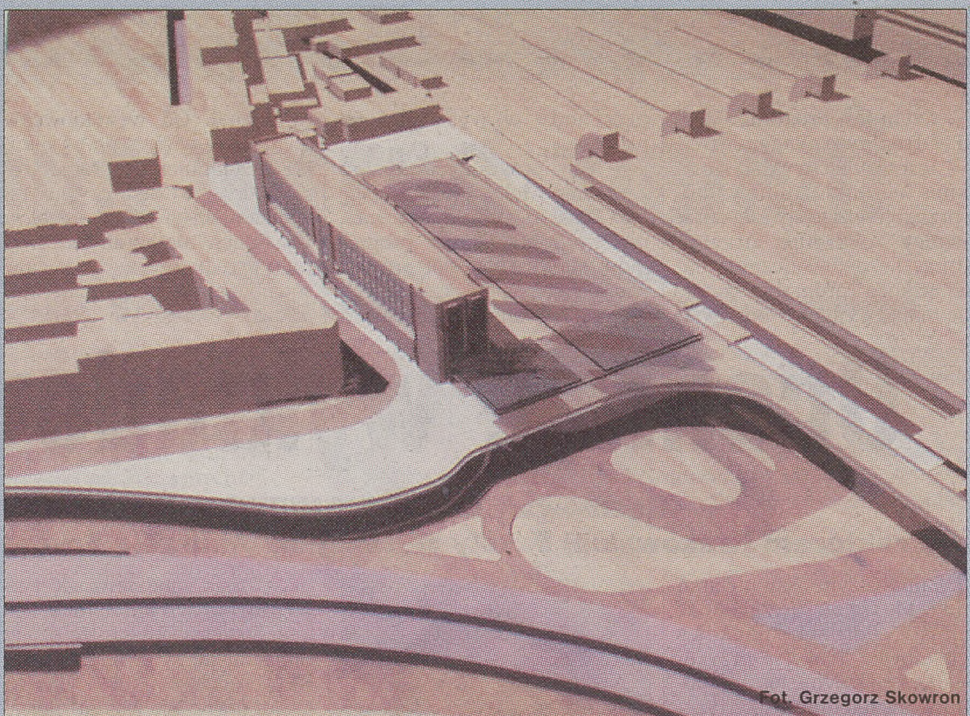
Koncepcja „Wasko”. Na dolnym poziomie będzie 26 stanowisk dla autobusów, a na górnym – 21 i 3 dodatkowe stanowiska dla wysiadających. Budynek dworca będzie miał ok. 1 tys. m kw. powierzchni użytkowej. Na każdy z poziomów będzie prowadził osobny wjazd. Szacunkowy koszt – ok. 14 mln zł.
