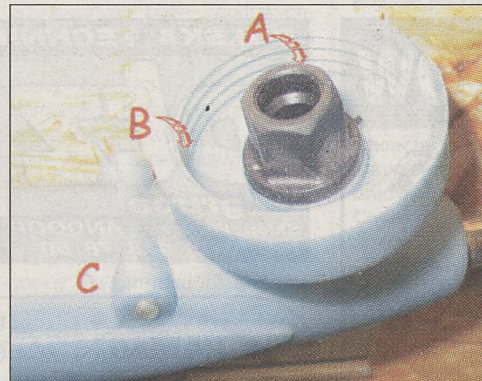
Tak wygląda głowica typu profi (A) pistoletu jednorazowego. Rękojeść wykonano z tworzywa sztucznego, z którego zaschniętą piankę usuwa się za pomocą cienkiego patyczka, gdyż się do niego nie klei. Mimo że jednorazowy – pistolet można rozkręcać (łącznik C).
