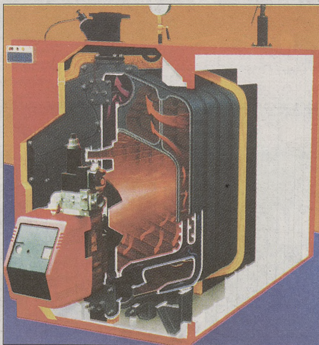
Wodny, niskotemperaturowy kocioł olejowo-gazowy
