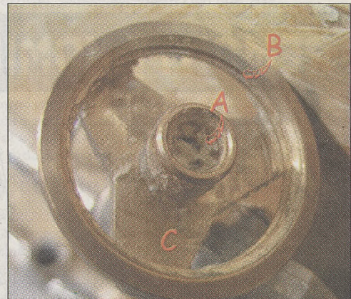
Oto głowica bardzo zaniedbanego pistoletu profesjonalnego (mocowanie typu rondel). Najważniejsze przy jej czyszczeniu jest udrożnienie wnętrza (A). Po wykręceniu pianki resztki zawsze należy wybrać ze środka za pomocą plastikowej nakładki ze specjalnym występem, która jest na butli. Jeśli pianka jest tak zaschnięta jak na zdjęciu, miejsce A trzeba zalać płynem czyszczącym, odczekać i starannie wyskrobać drewnianym, aby dotrzeć do kulki z tworzywa, następnie ponownie zalać płynem i tak długo trzymać, aż uda się za pomocą zapalki nacisnąć na kulkę – tak, aby się poruszyła (jest na sprężynce). Ta kulka to zawór i musi swobodnie się poruszać. Strefa C powinna być w miarę czysta, ale gwint (B) musi być sterylny, gdyż ma prawidłowo trzymać wkręcaną butlę.
