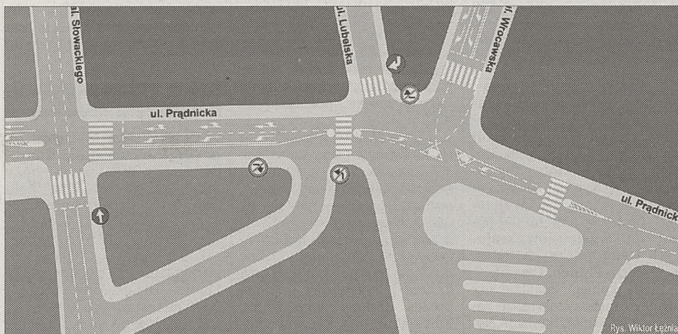
Projekt uporządkowania ruchu na skrzyżowaniu
