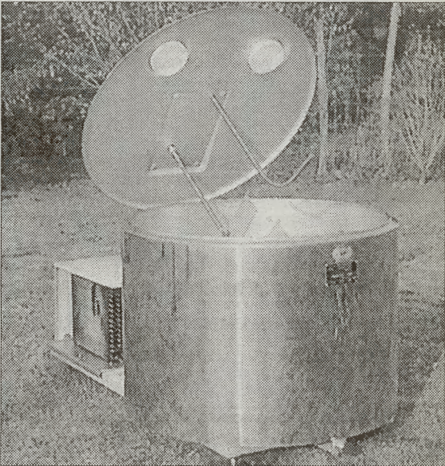
Schładzalnik cylindryczny pionowy o pojemności od 100 do 1950 l mleka
