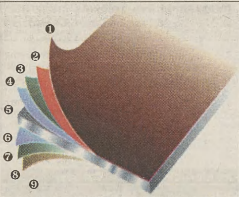
1 - kolorowa powłoka zewnętrzna, 2 - podkład, 3 - warstwa pasywna, 4 - cynk, 5 - blacha stalowa, 6 - cynk, 7 - warstwa pasywacyjna, 8 - podkład, 9 - powłoka ochronna
