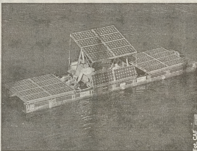
Łódź „Karin” w porcie w Sydney – to największa łódź o napędzie wykorzystującym energię słoneczną. 28 paneli słonecznych umożliwi podróżowanie na długich dystansach
