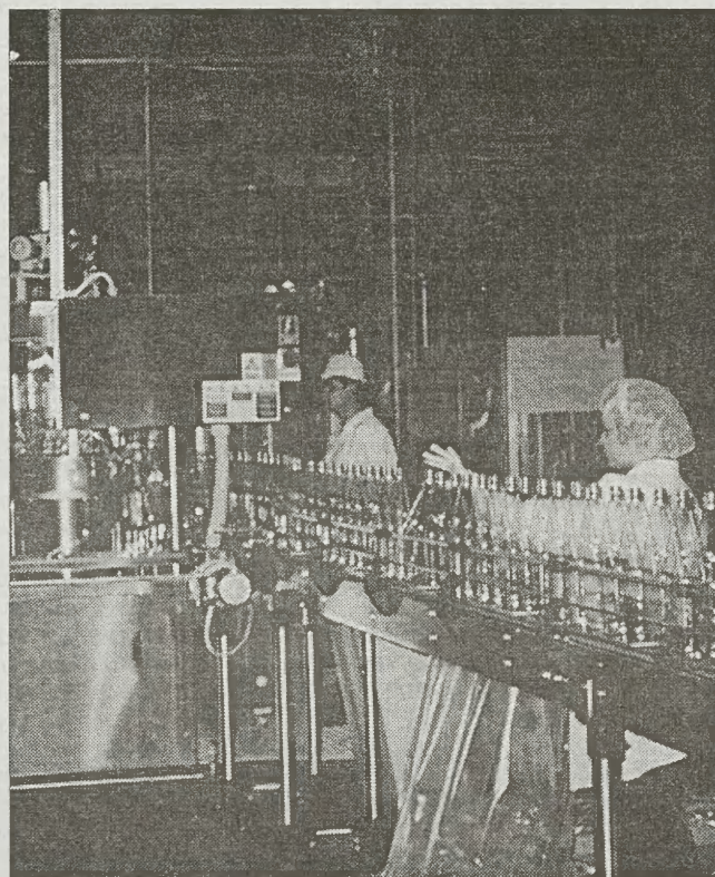
Najnowsza inwestycja Tymbarku — nowoczesna linia do rozlewu wody mineralnej o wydajności 80 tys. butelek na dobę
