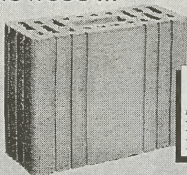
CEGLA MODULARNA Z UCHWYTEM kl. 150 zastosowanie: - ścianki działowe - ściany warstwowe, zewnętrzne - ściany osłonowe - ściany wypełniające
