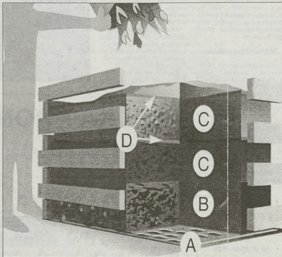
(A) – dno nie jest konieczne, jeżeli zostanie zastosowane, musi umożliwiać przechodzenie małych żyjótek (B) – warstwa materiału gruboziarnistego, umożliwiającego krążenie powietrza (C) – warstwy zawierające zrównoważony stosunek azotu do węgla (D) – cienka warstwa ziemi lub kompostu
