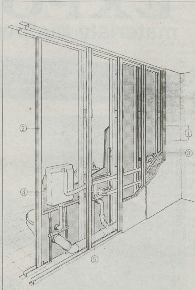
Na lekkich ścianach z płyt kartonowo-gipsowych można wieszac ciężkie przedmioty, m.in. umywalkę, sedes 1. płyta kartonowo-gipsowa 2. metalowa konstrukcja nośna 3. wełna mineralna 4. stelaż ze spluczką WC 5. stelaż pod umywalkę
